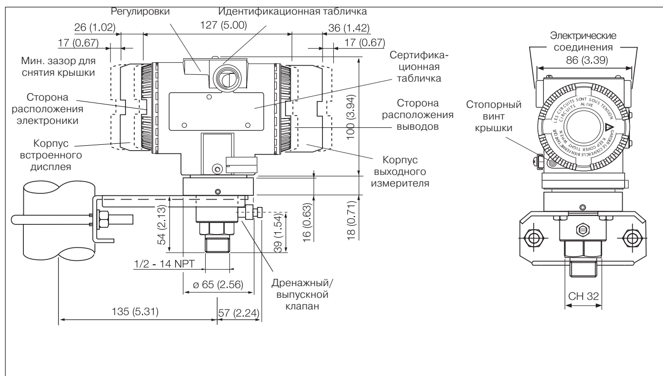
Соединение с внешней резьбой 1/2 - 14 NPT
