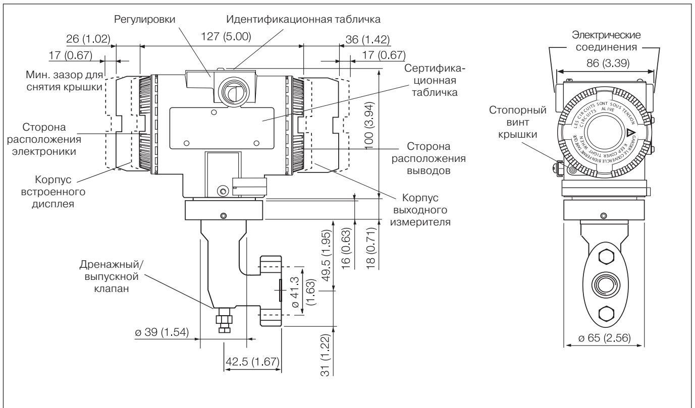
Адаптер с угловым входным (90°) соединением (сверление \frac{7}{16} – 20 UNF)
