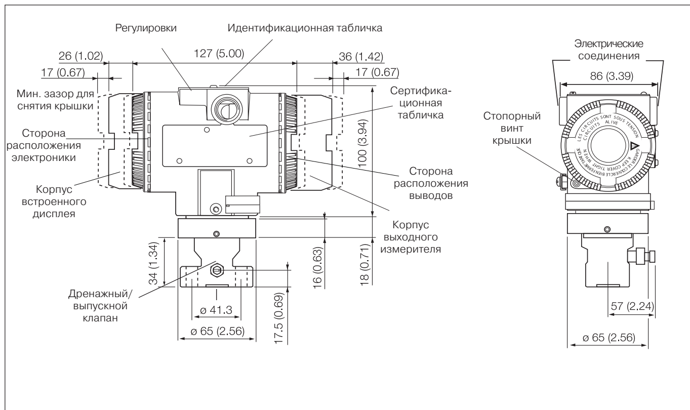
Адаптер с прямым входным (180°) соединением (сверление 7/16 - 20 UNF)
