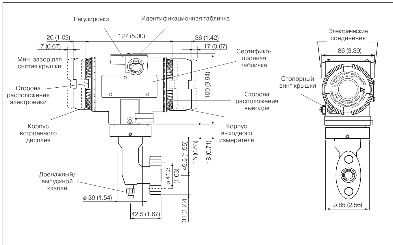
Адаптер с угловым входным ( 90^\circ ) соединением (сверление 7/16 - 20 UNF) для сенсоров G, H, M, P, Q, S
