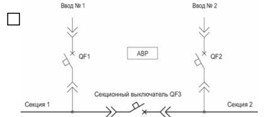
Два рабочих ввода на шину с секционированием
