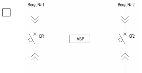
Два рабочих ввода на общую шину
